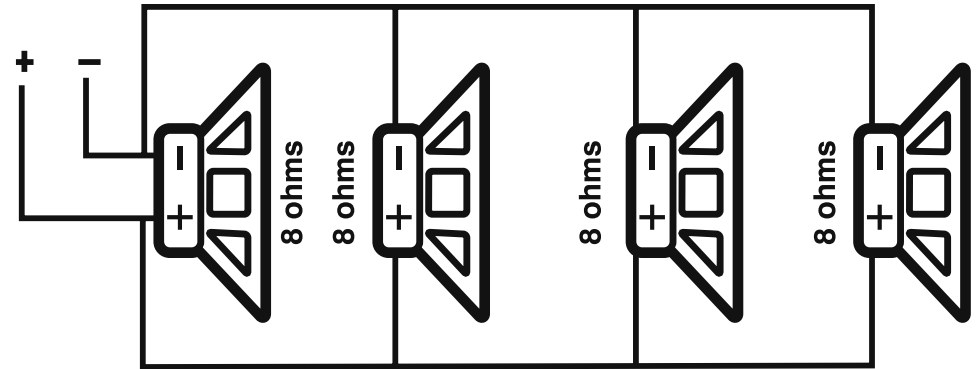
B: PARALELO 2 ohms
