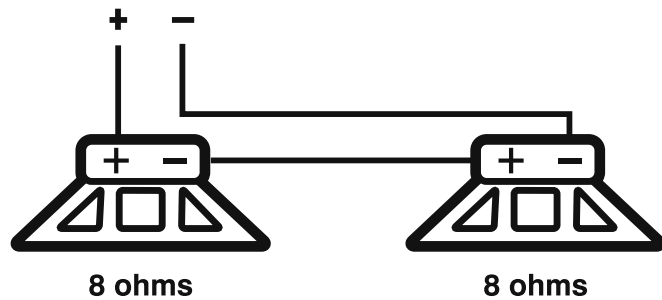
C: SERIE 16 ohms
