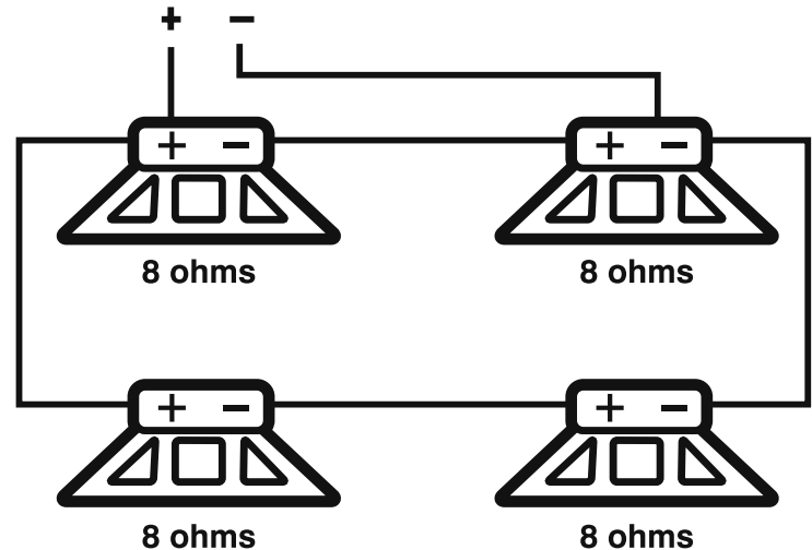
D: SERIE PARALELO 8 ohms
