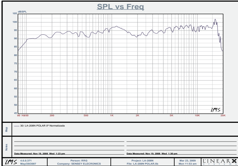
Gráfica SPL, 1W, 1 mt, Unidad.
