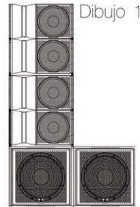
2. Arreglo lineal monofónico (dibujo 1).
